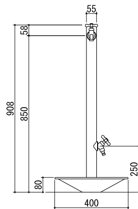
立面図
