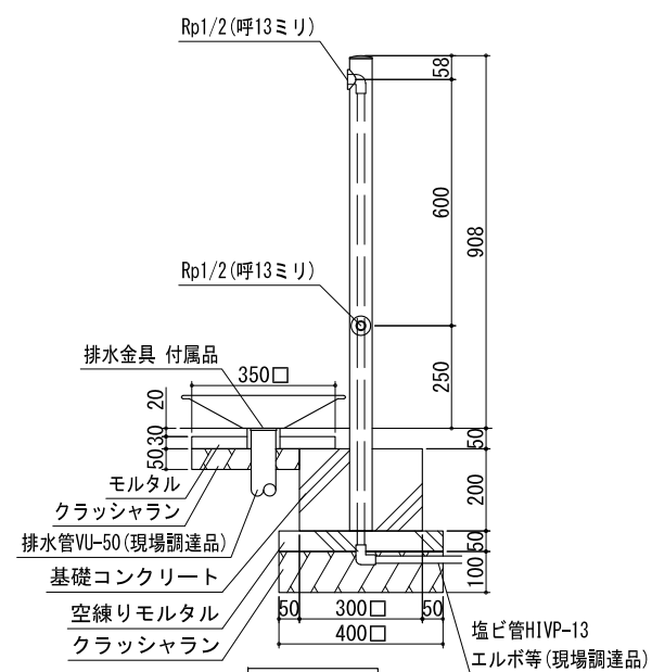
側断面図
