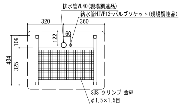
A-A断面・給排水管位置図
