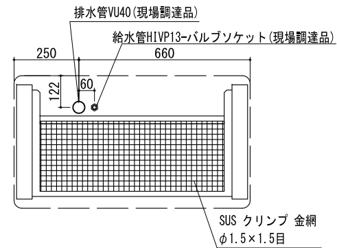
A-A断面・給排水管位置図
