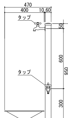
側面図
