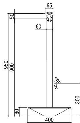
立面図
