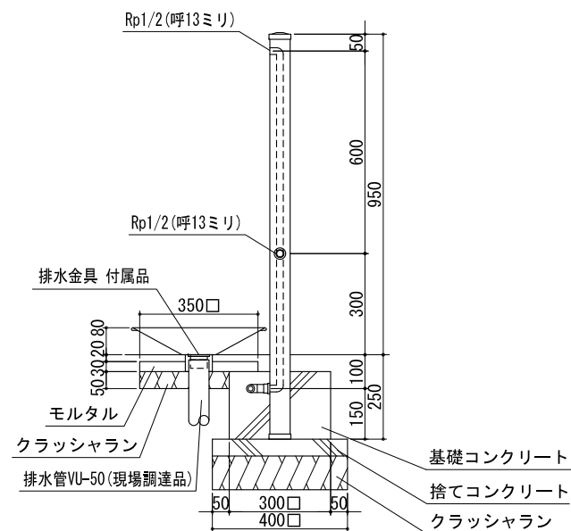
側断面図
