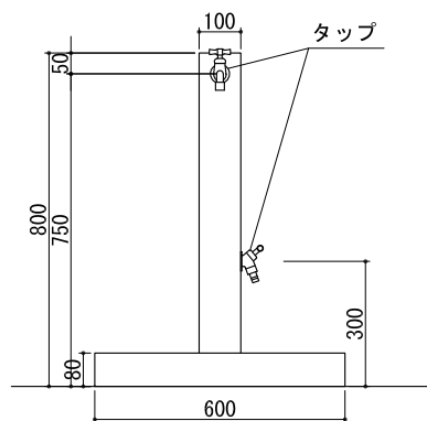
立面図
