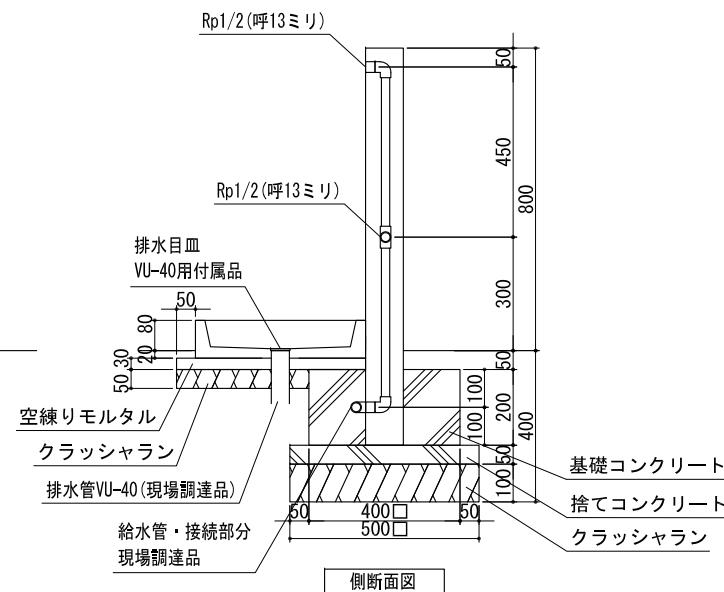
側断面図
