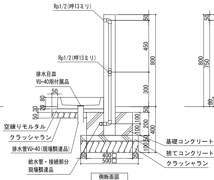
側断面図
