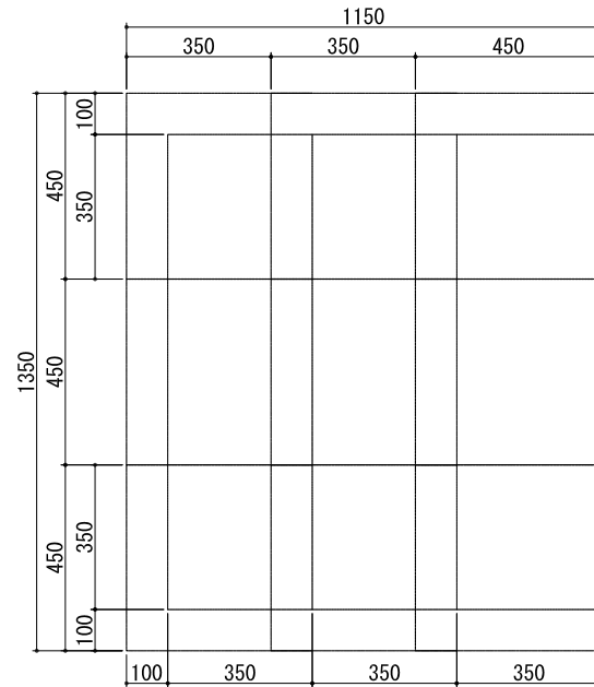
蹴込み寸法100mm以下のとき
