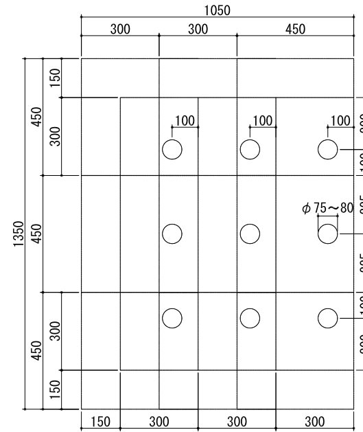
蹴込み寸法101~150mmのとき
