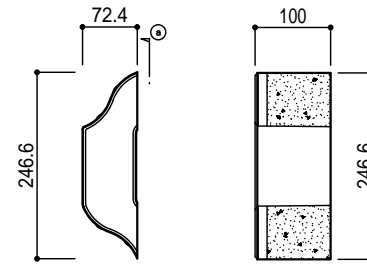
a 断面図
