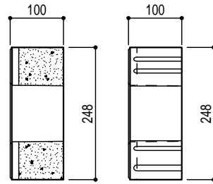
a 断面図
