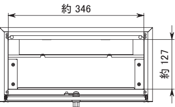
▼ 後面図(全開) 投入口寸法
