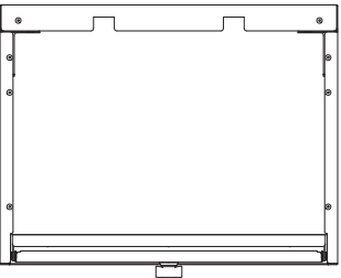
▼ 後面図(全開) 投入口寸法
