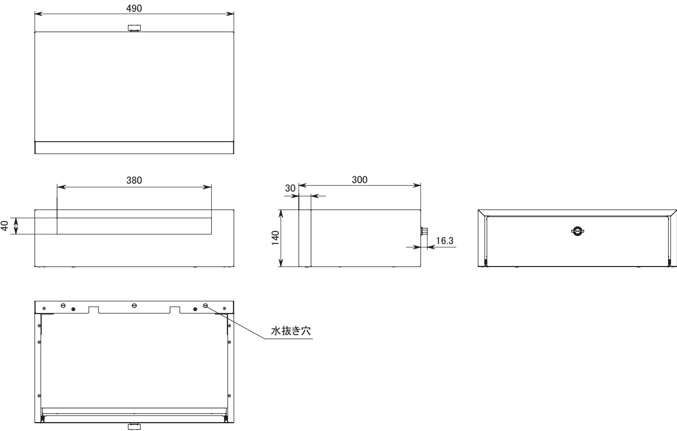
▼ 後面図(全開) 投入口寸法
