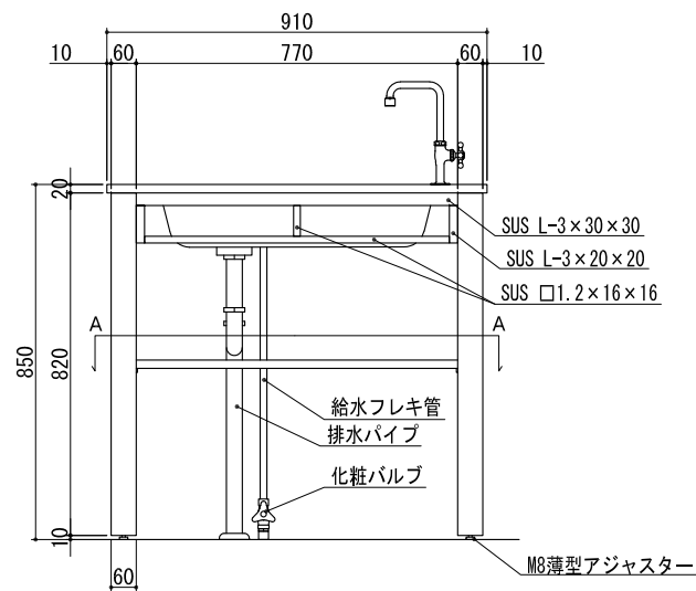
正面図
