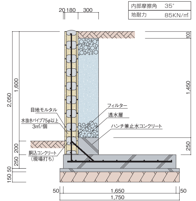
TY 型枠ブロック プレーン 180 型
